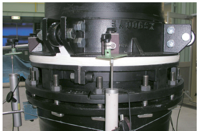
●NS形EPSリングの圧壊試験状況
